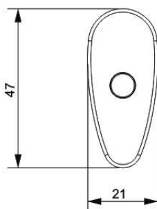
Závaží Duo rolety s ložiskem
