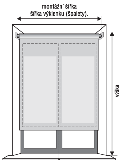
roleta v okenním výklenku (ve špaletě) šířka výklenku (špalety) = mont. šířka
