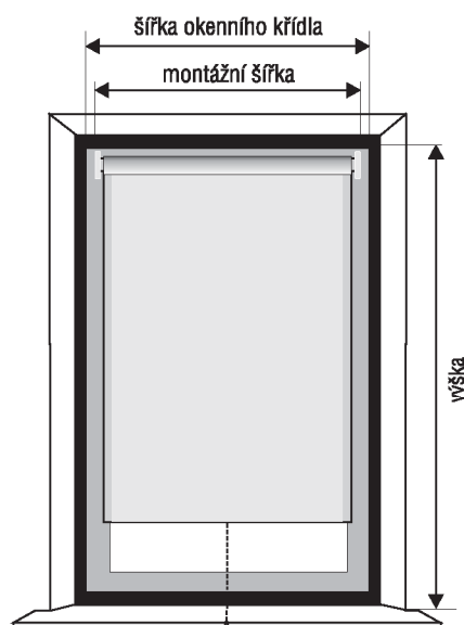
roleta na okenním křídle od okenního křídla odečtete cca 2cm = mont. šířka
