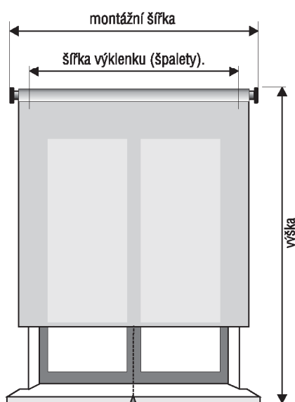
roleta před okenním výklenkem k šířce výklenku přičíst min. 11 cm = mont. šířka
