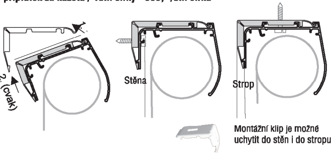
Obr. 1 Otevřená roleta
