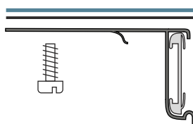
Montáž na strop
