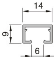
průřez kolejničkou
