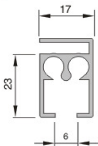
průřez kolejničkou
