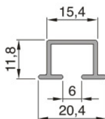
průřez kolejničkou
