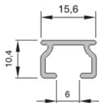
průřez kolejničkou
