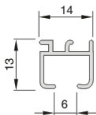
průřez kolejničkou
