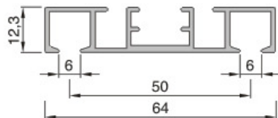
průřez kolejničkou
