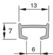
průřez kolejničkou
